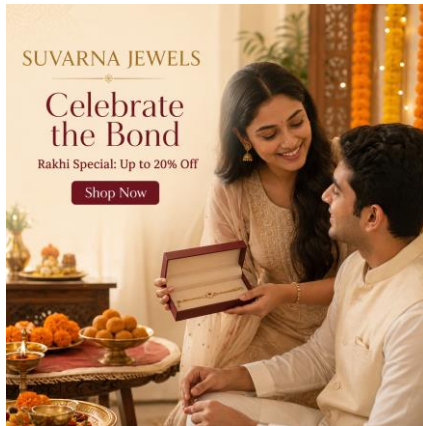
GPT
